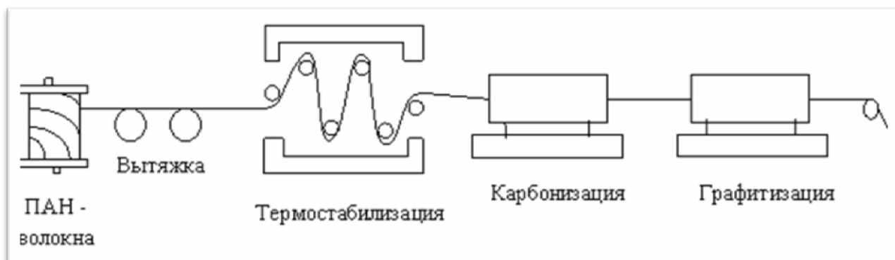
а) Схема получения углеродного волокна из ПАА-волокон
