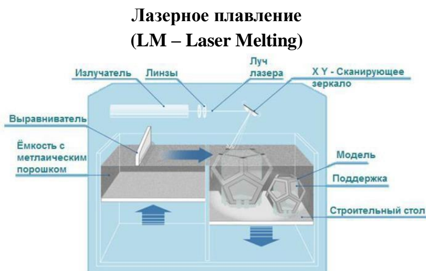
Рисунок 42 – Схема процесса LM
